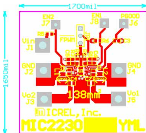
Top Layer
